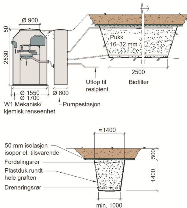
Tverrsnitt av biofilter
